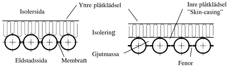
Fig 24. Membranvägg.
