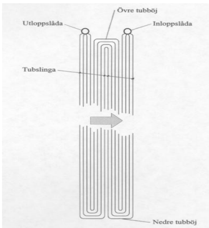
Fig. 9. Överhettarskärm.
