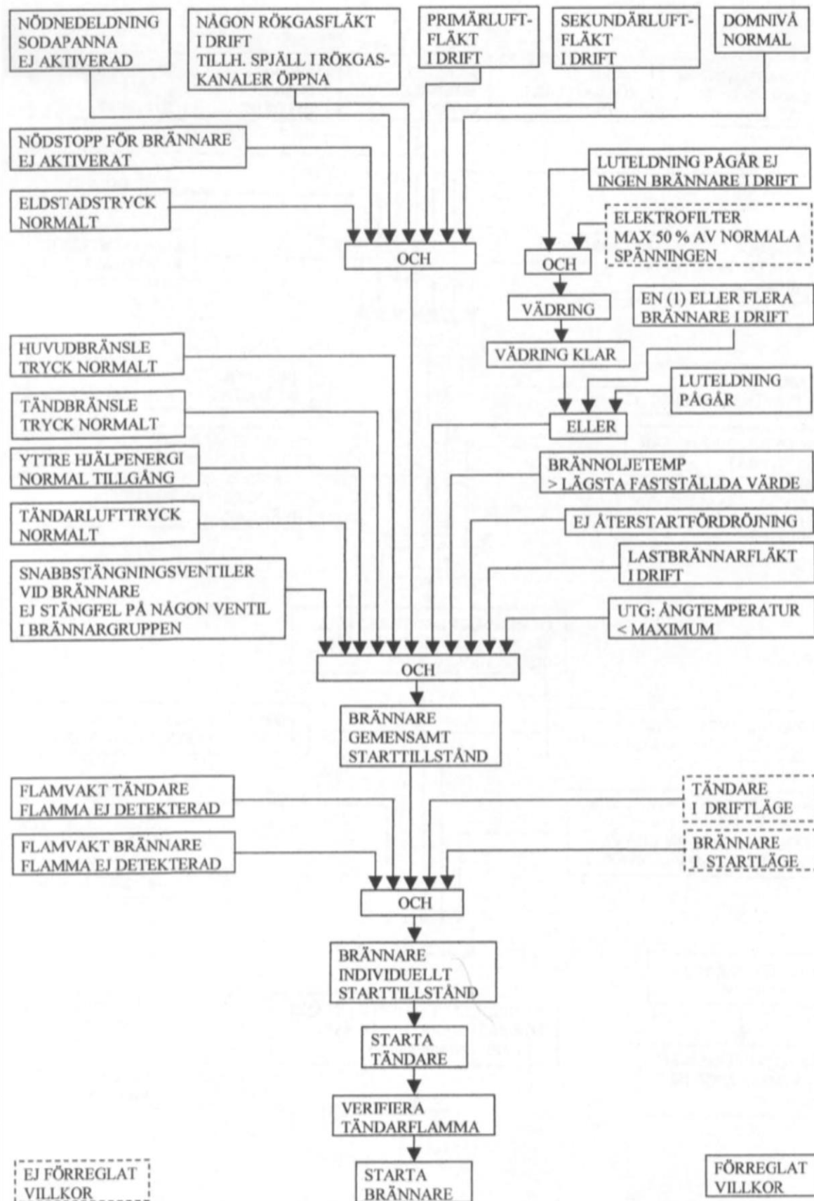
Figur 2, Exempel på startvillkor för oljeeldade lastbrännare
