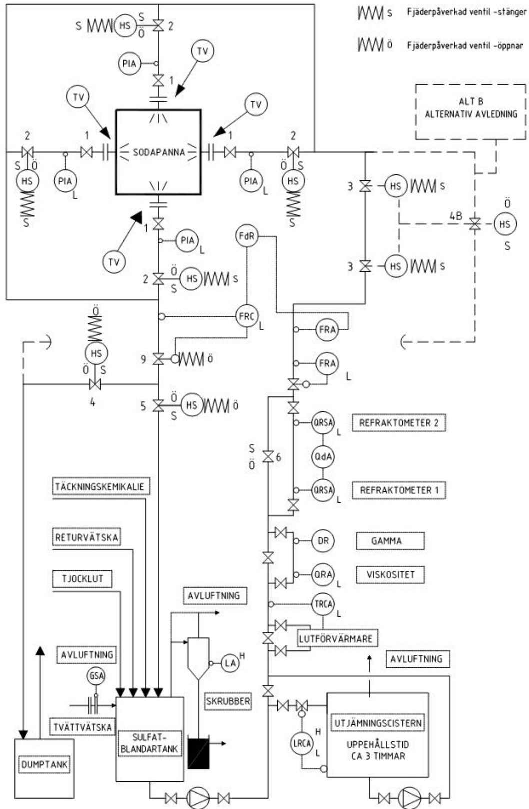
Figur 1, Lutsystem anslutet till öppen (inte trycksatt) cistern och med system för avledning till dumptank
