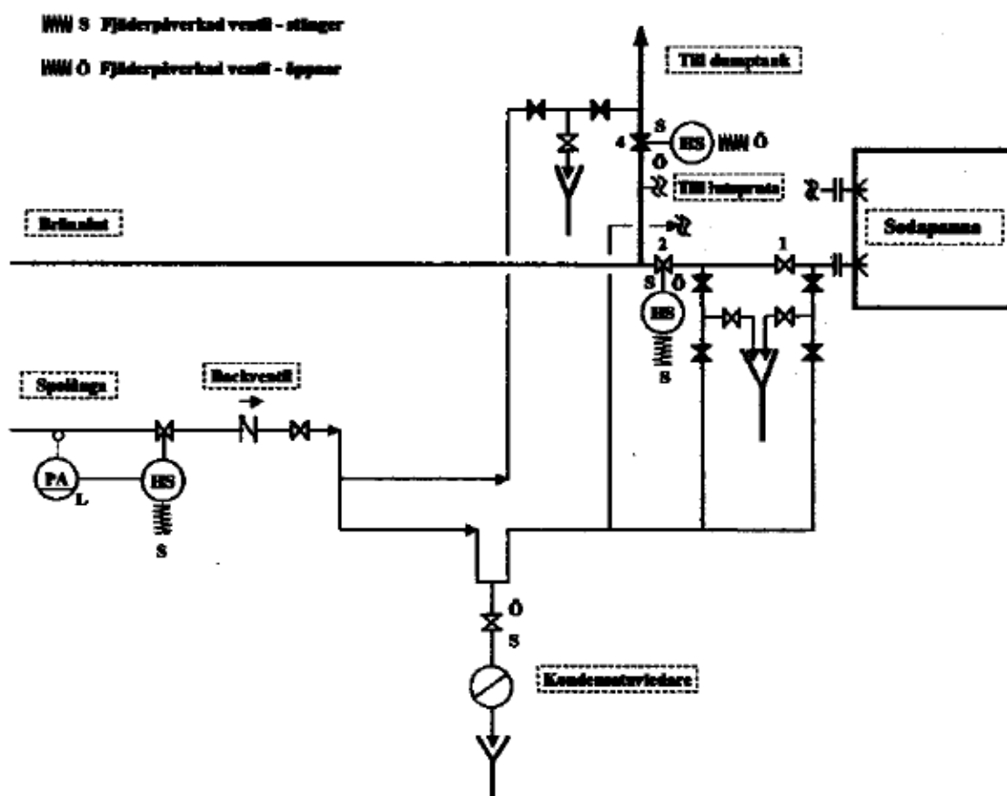
Figur 4, Arrangemang vid ångblåsning av brännlutlutledningar
