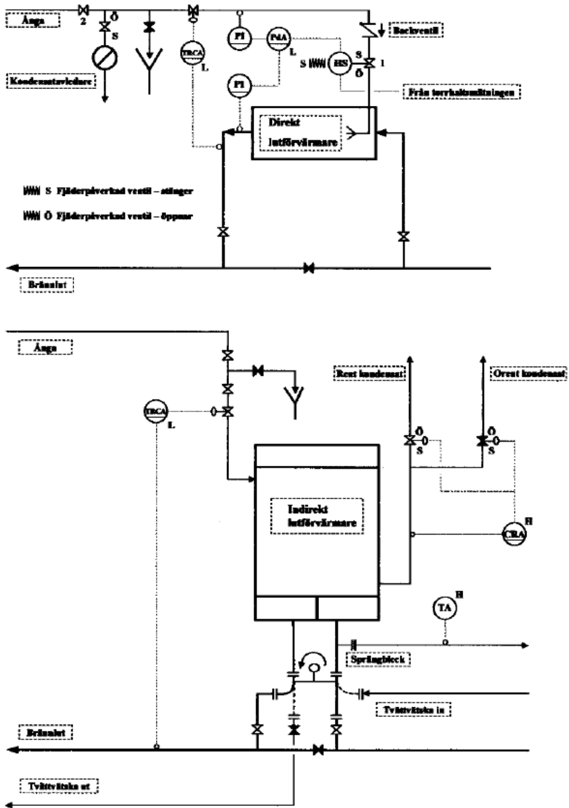
Figur 3, Arrangemang vid direkt respektive indirekt luftförvärmare
