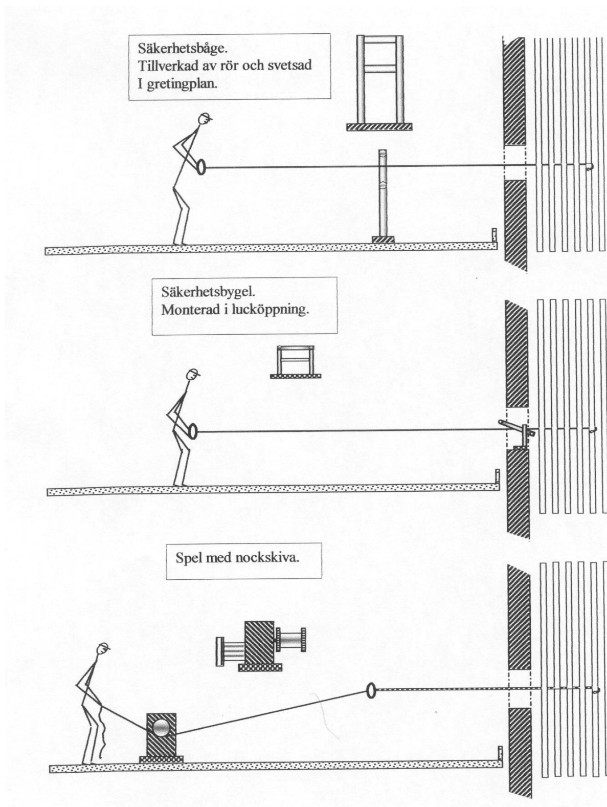
Figur 1, Exempel på arrangemang för handlansning av överhettare
