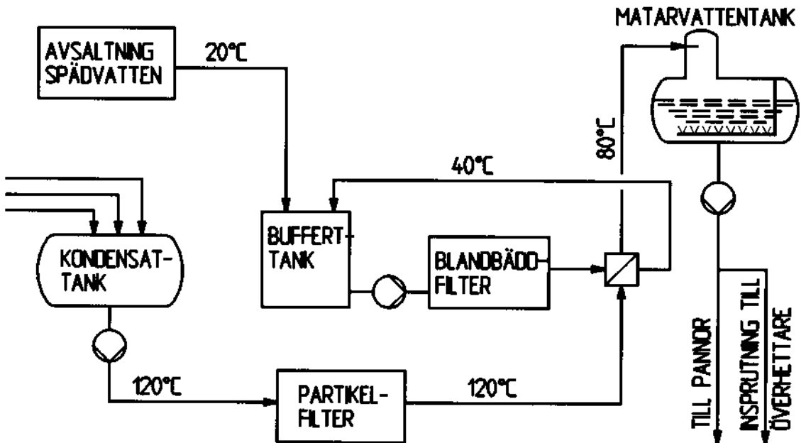
Fig. 2. Blandbäddfiltrerat matarvatten
